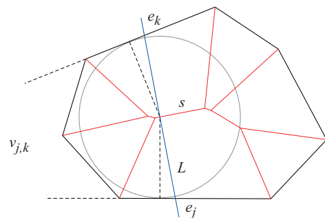
Figure 5: Lemma 4.
